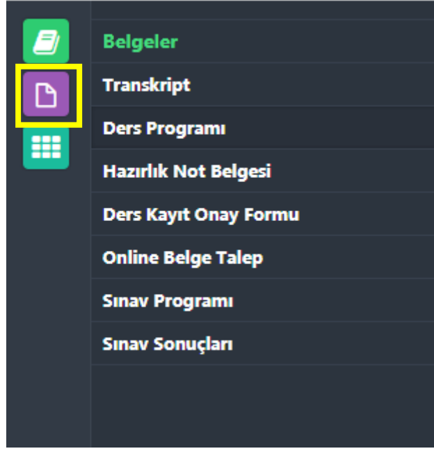
Şekil 6 Belgeler Menüsü
