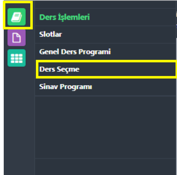
Şekil 5. Ders Seçimi
